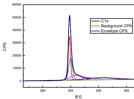
小尺寸石墨烯 XPS 图谱及拉曼图谱。小尺寸石墨烯内部结构完整，边缘丰富且存在缺陷，便于改性。
