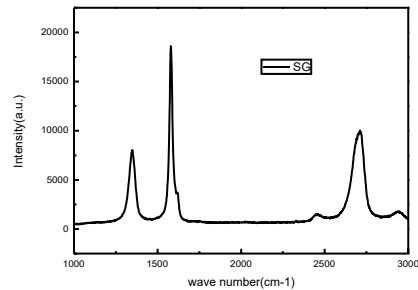
小尺寸石墨烯 XPS 图谱及拉曼图谱。小尺寸石墨烯内部结构完整，边缘丰富且存在缺陷，便于改性。
